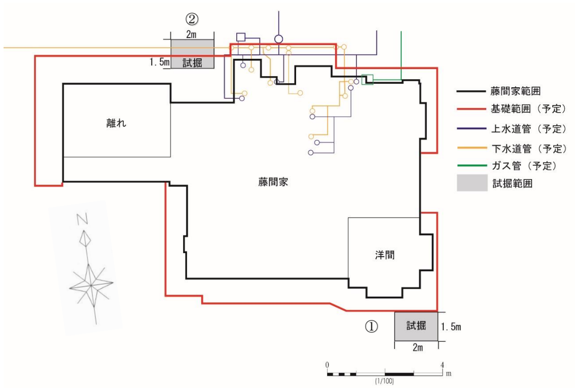
図3 調査区配置図 (案)
