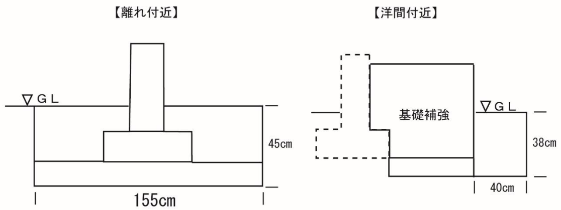
図4 基礎断面図 (案)
