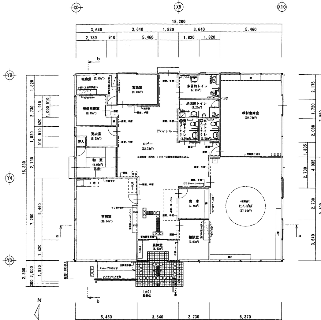
平面図 1/100
