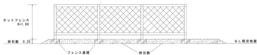
図3 砕石盛土・ネットフェンス概念図工事地点近景（上が北）
