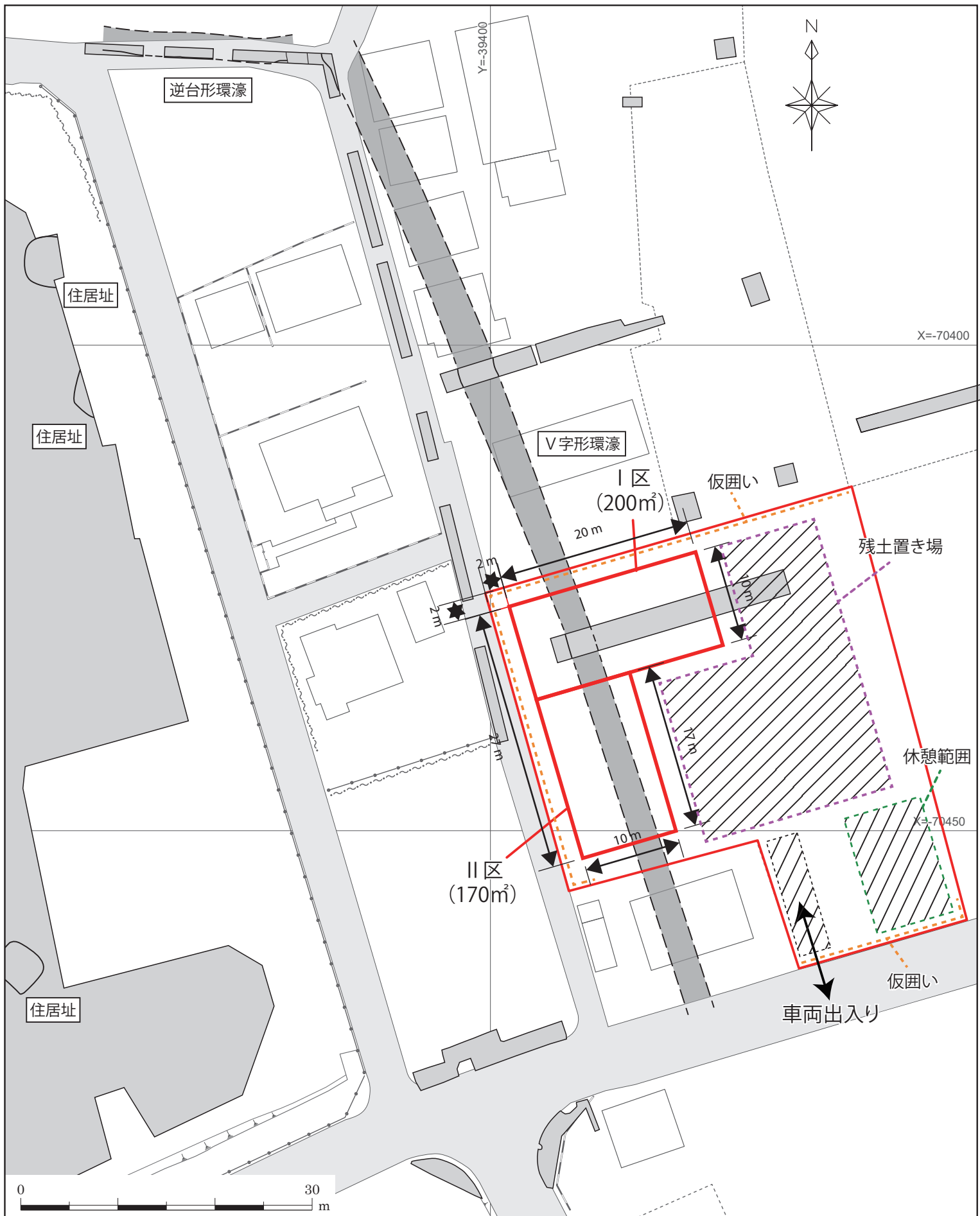
第4図 調査計画図（史跡下寺尾西方遺跡）
