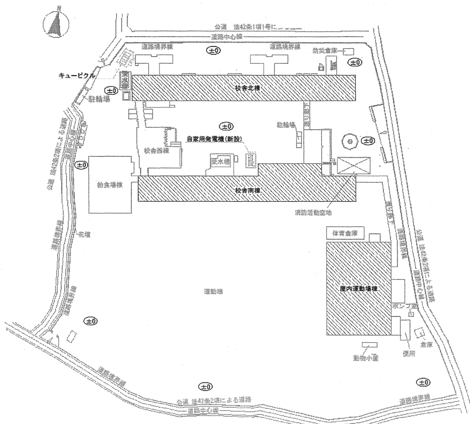
配置図
