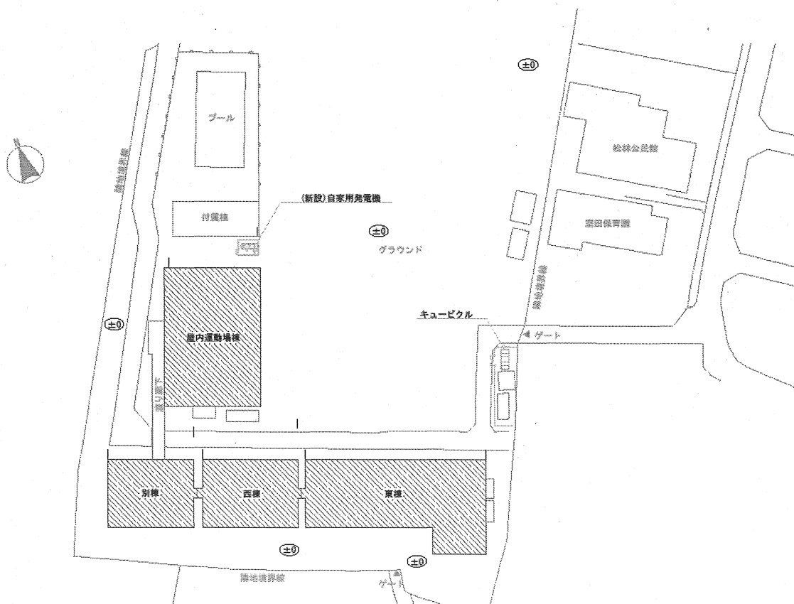
配置図
