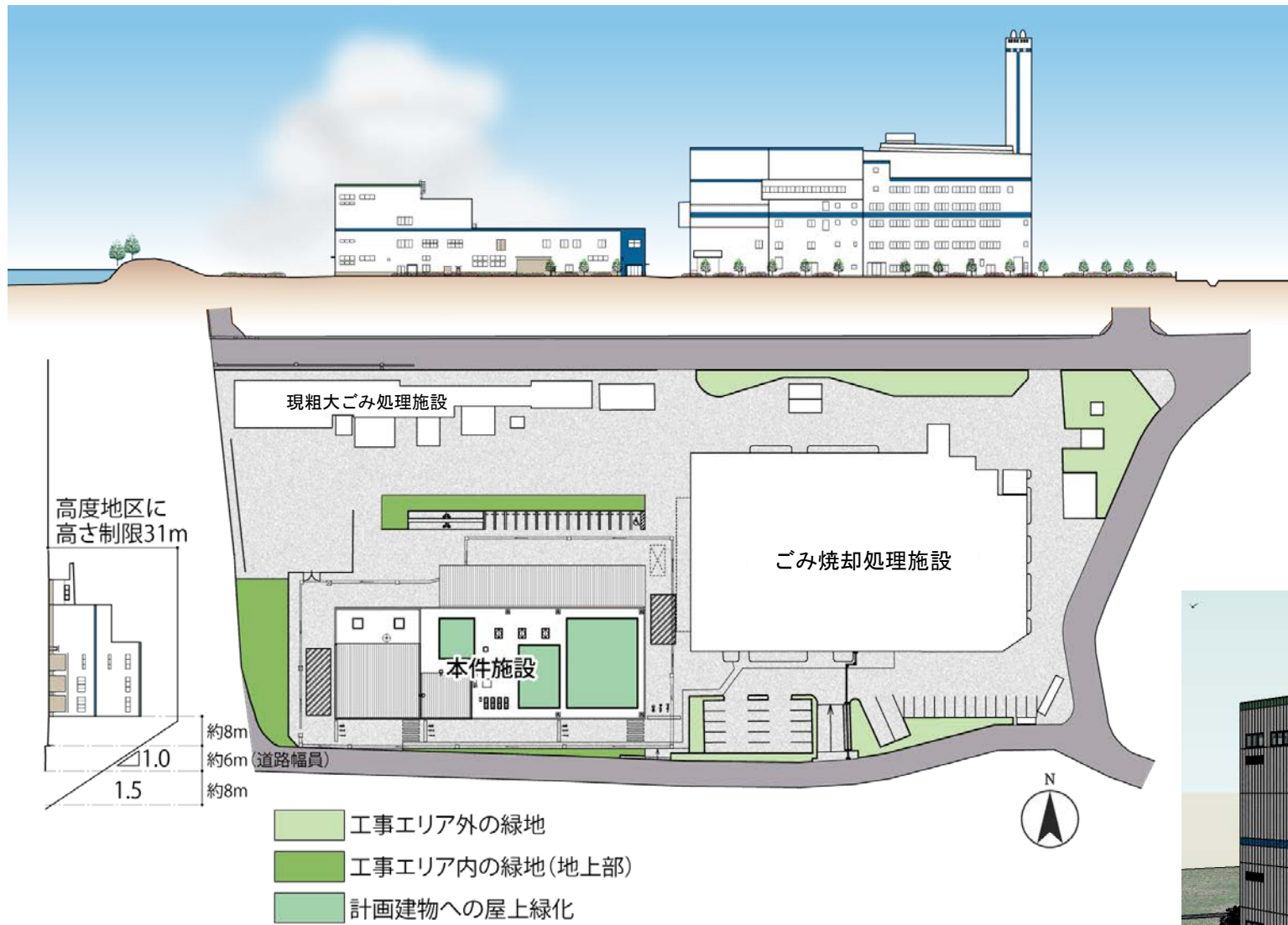
配置図・立面図
