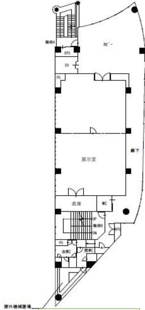
4階平面図
