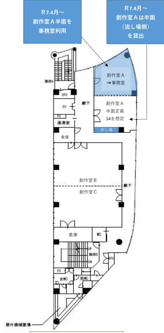
5階平面図
