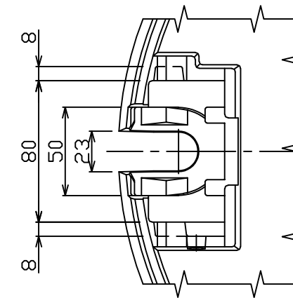
シールロック取付座詳細図
