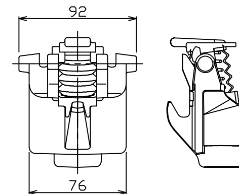
シールロック詳細図
