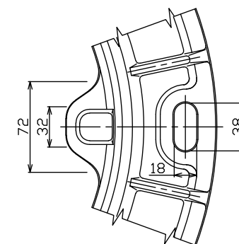
コネクタ受け部詳細図
