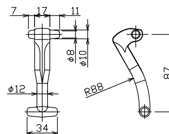
③ コネクタ詳細図
