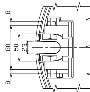
シーลロック取付座詳細図
