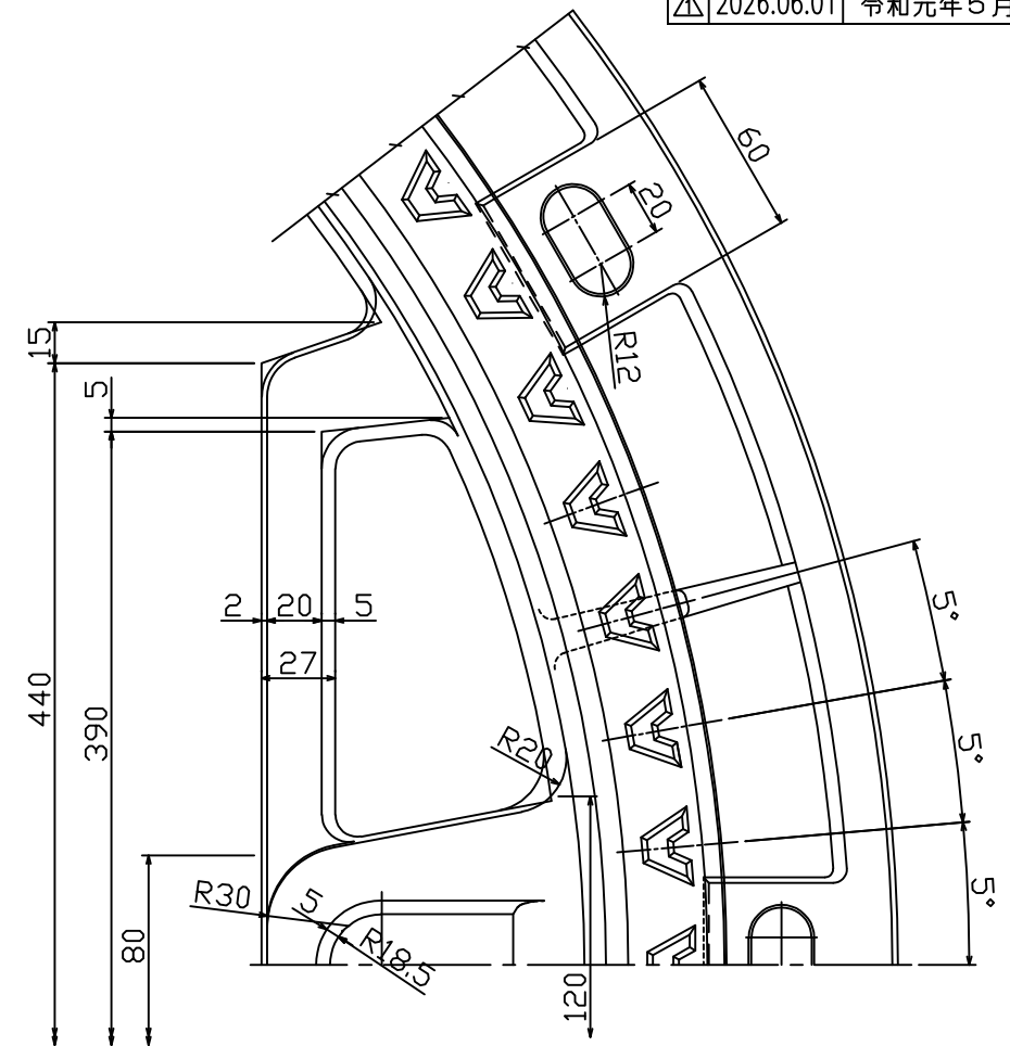
フレーム、コネクタ取付部詳細
