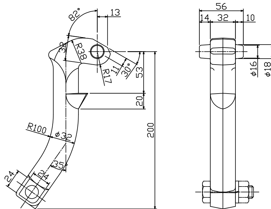
親蓋コネクタ詳細図
