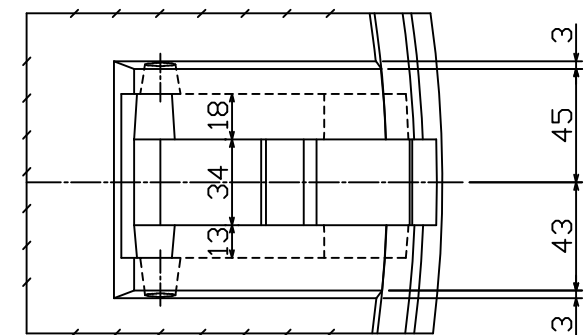
親蓋コネクタ取付座詳細図
