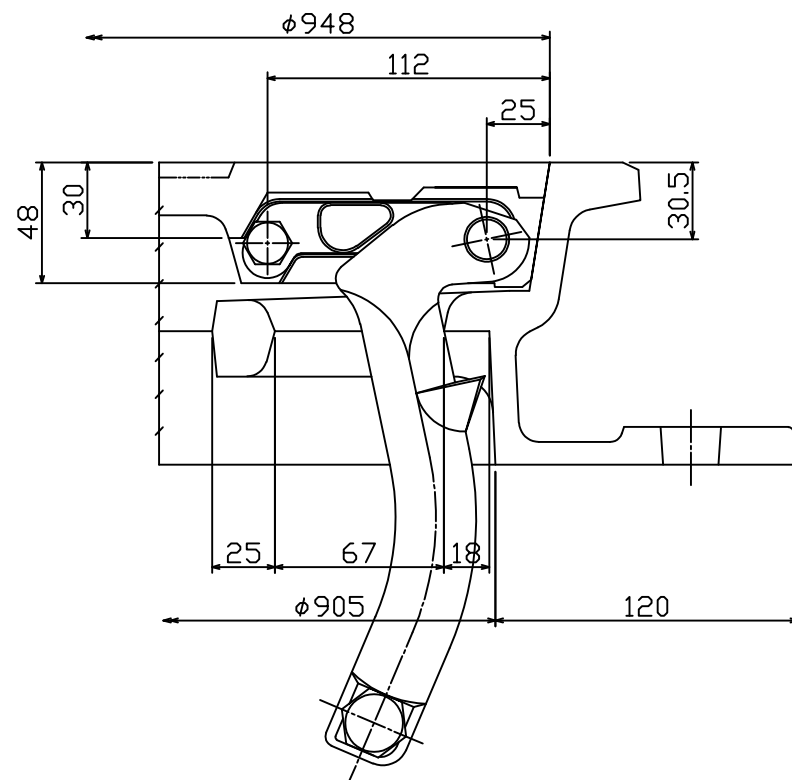
親蓋コネクタ取付部詳細図
