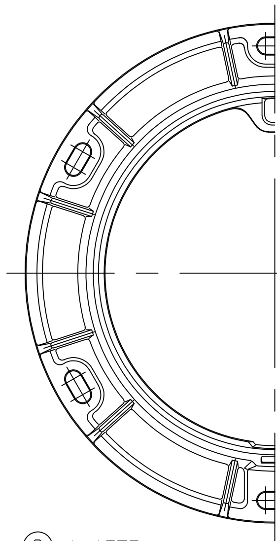
② フレーム平面図
