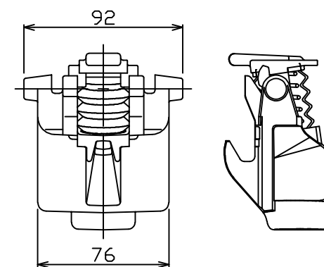
⑤ シールロック詳細図
