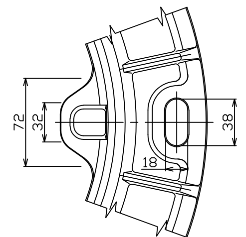
コネクタ受け部詳細図
