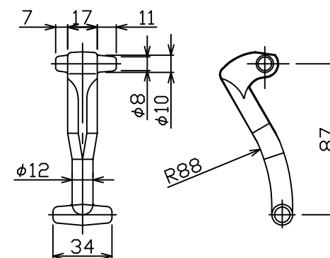
③ コネクタ詳細図
