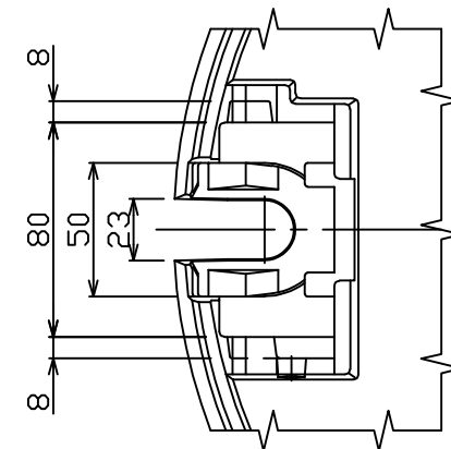
シーลロック取付座詳細図
