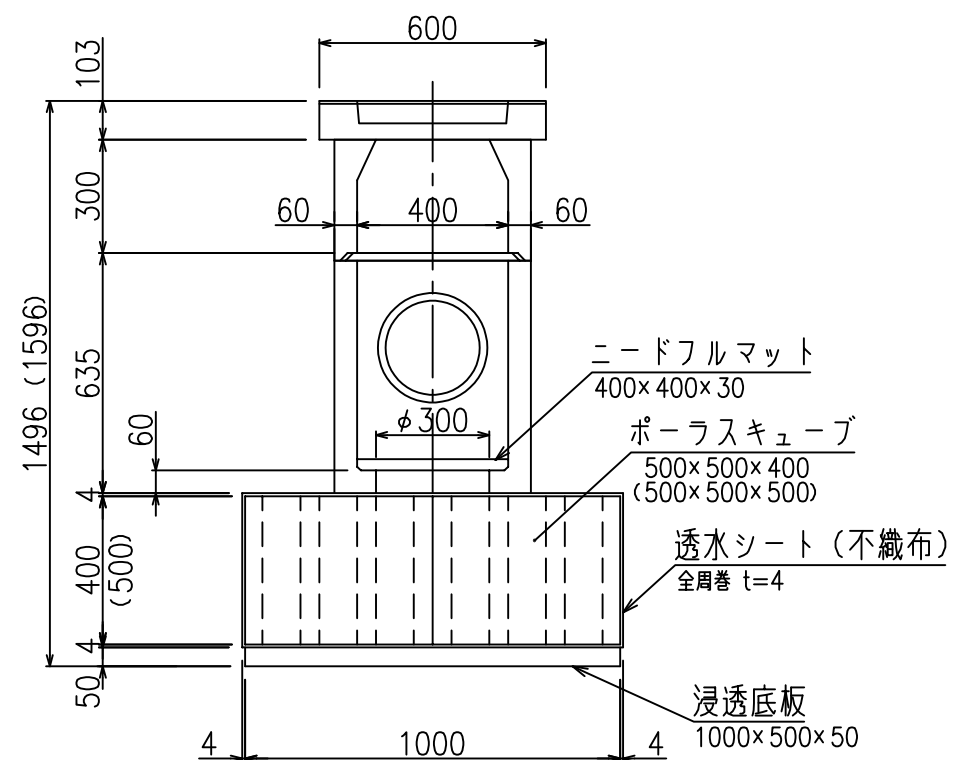
A-A 断面図
