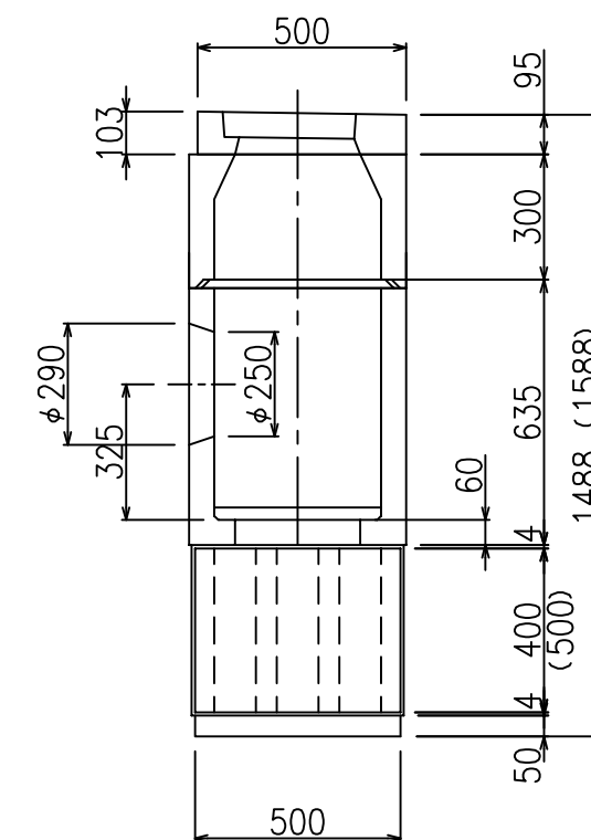
B-B 断面図
