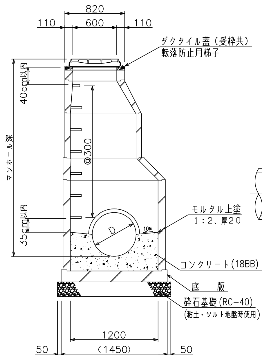
横断面図
