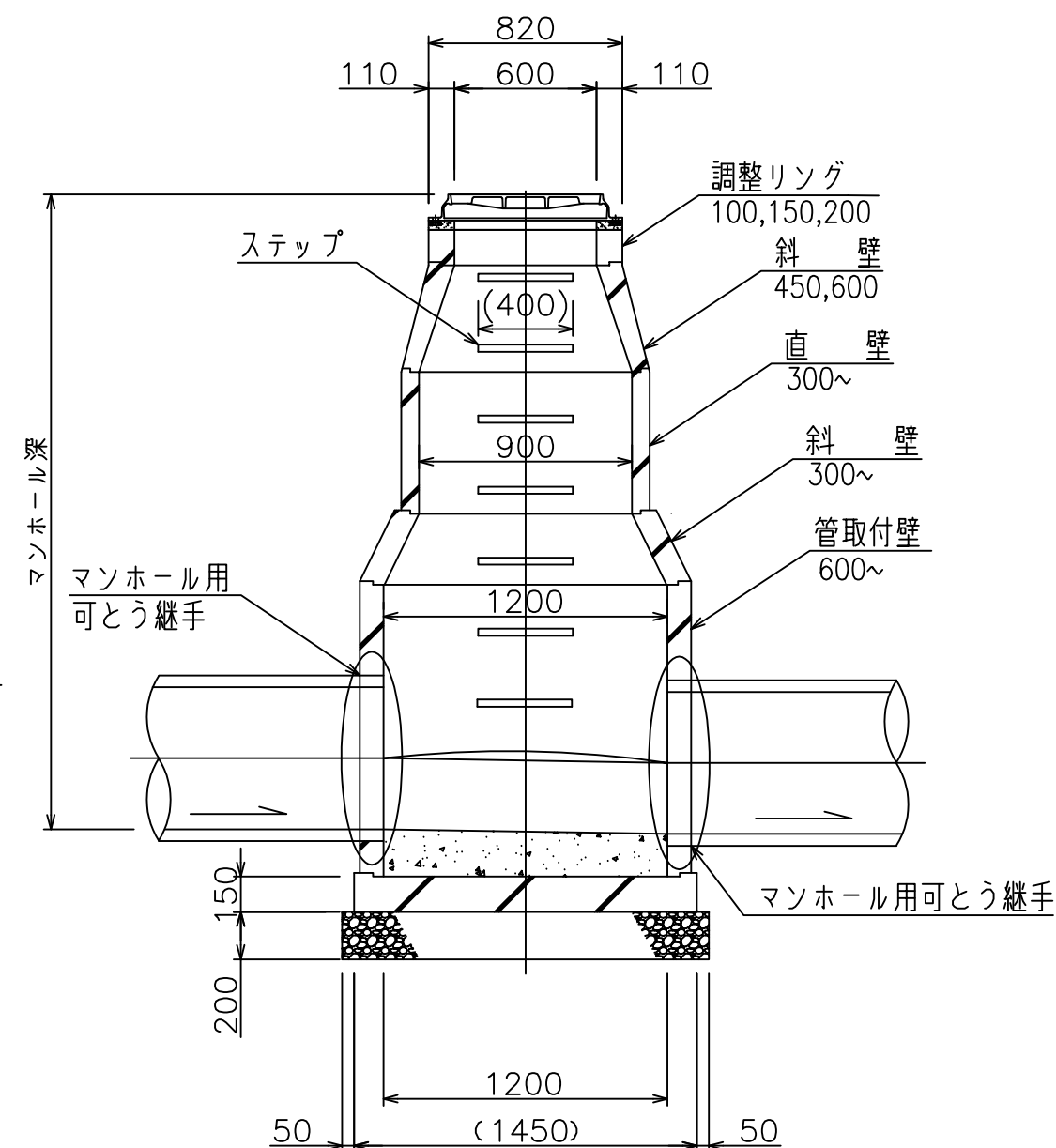
縦断面図
