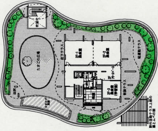
2階平面図
