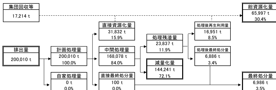
図-1 一般廃棄物（ごみ）の処理状況フロー（令和２年度）
