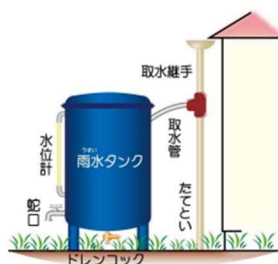
図 4.3 雨水貯留タンクのイメージ
