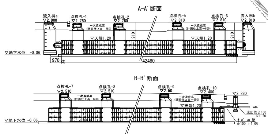
雨水貯留施設断面図
