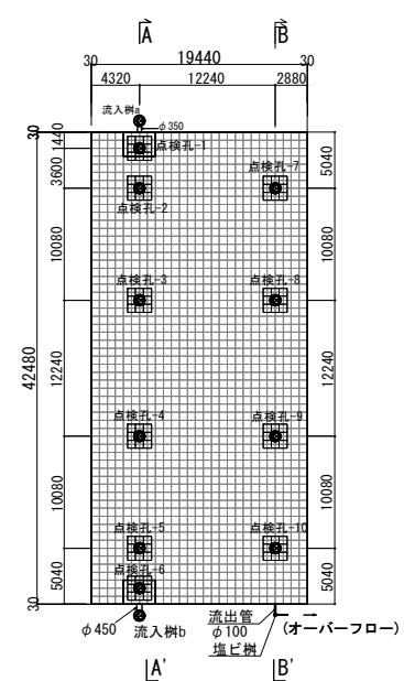
雨水貯留施設平面図
