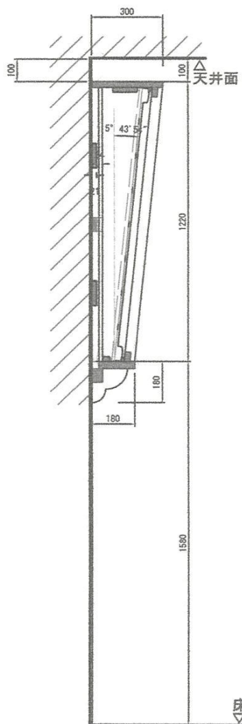
絵馬 断面図 S=1:20
