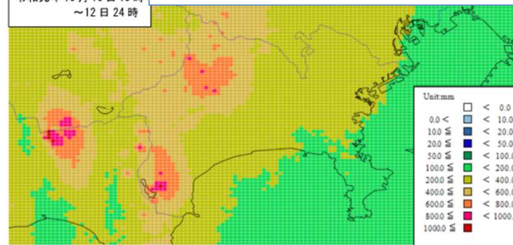
解析雨量による降水分布図
