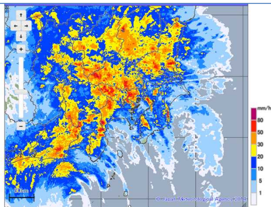
高解像度降水ナウキャスト 2019.10.12 15時30分
