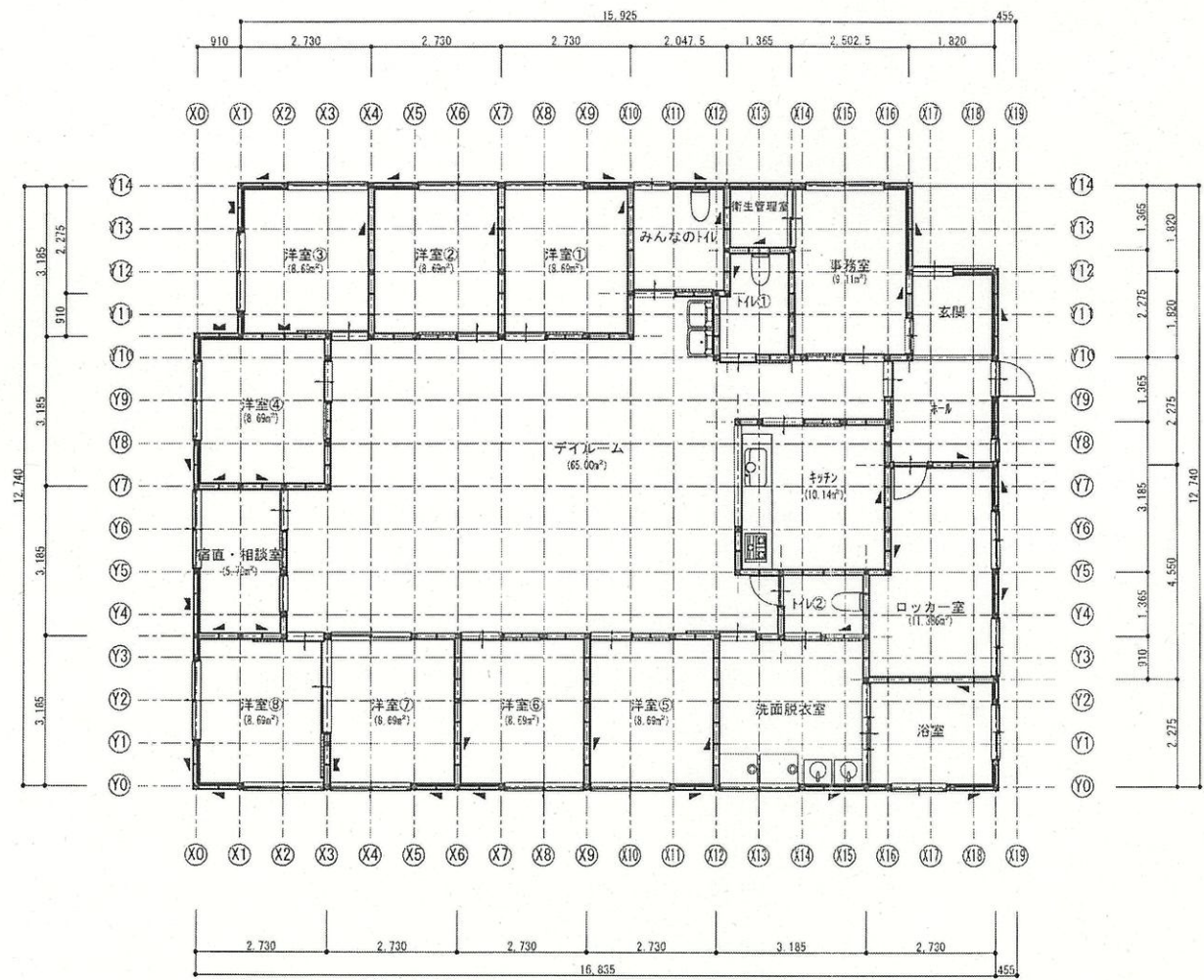
一階平面図 S=1:100
