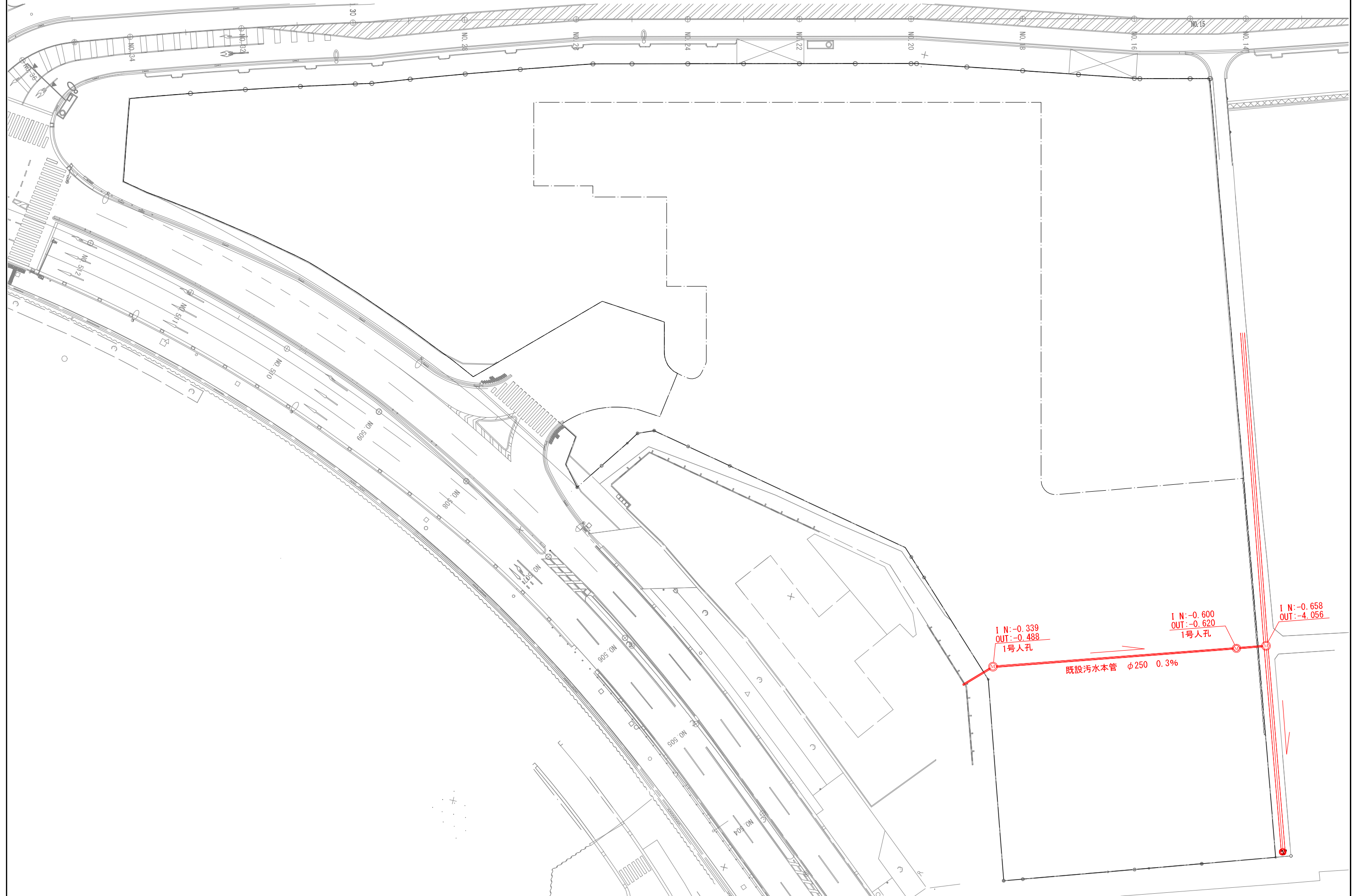
污水管整備状況図 S=1:600
