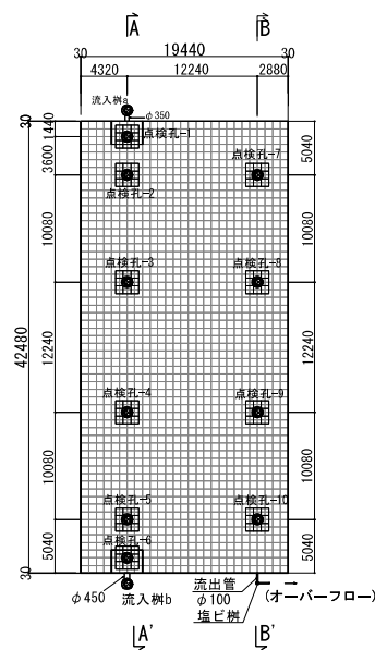
雨水貯留施設平面図
