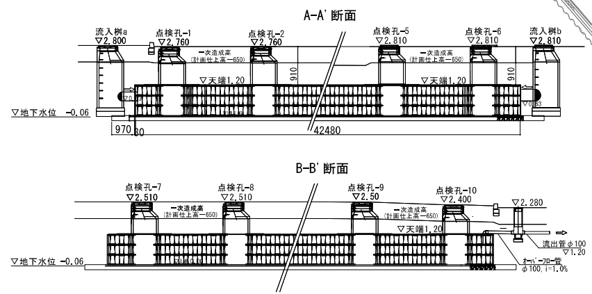
雨水貯留施設断面図
