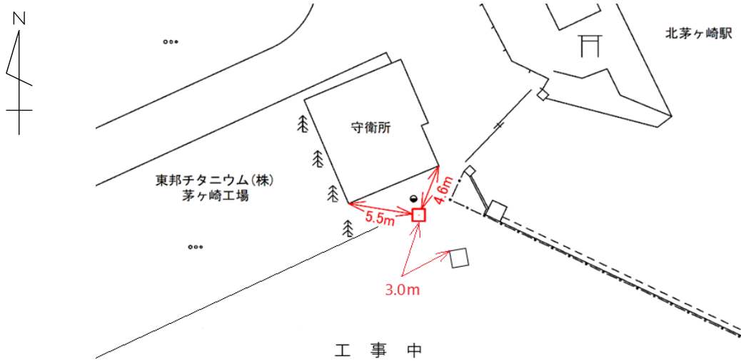
水準点詳細図
