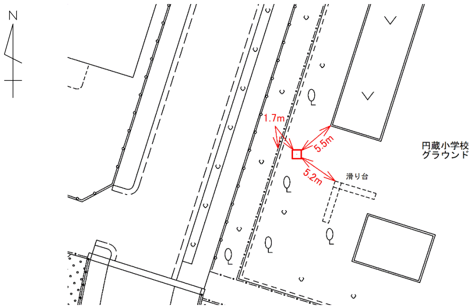
水準点詳細図
