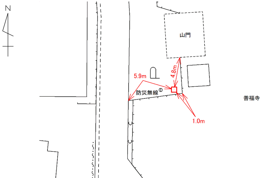
水準点詳細図
