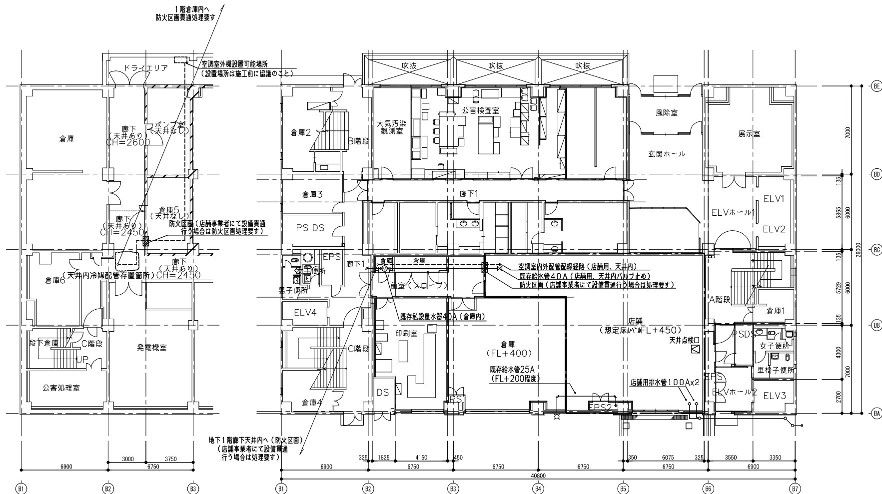
分庁舎 地下1階平面図
